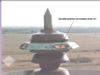
PARAFULMINE (PARTICOLARE) Foto di: ARPA Friuli Venezia Giulia Radionuclide: Am-241 Provenienza:
